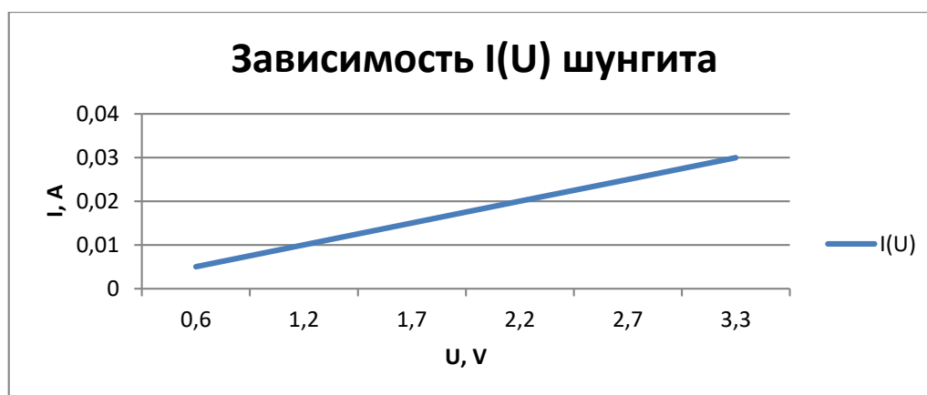
Рисунок 1 - Зависимость приложенного тока к 1 и 4 электродам от напряжения на 2 и 3 электродах (шунгит)
