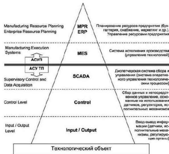
Рисунок 2 - Схема уровней и систем автоматизации
