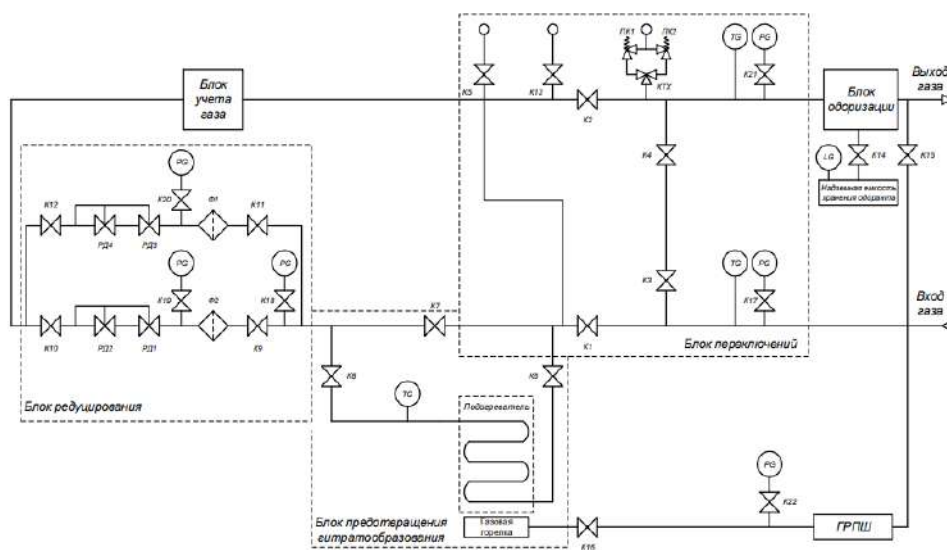
Рисунок 1 - Технологическая схема ГРС-10
