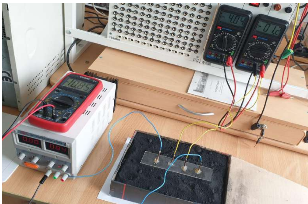
Рисунок 1 - Установка для измерения удельного сопротивления
