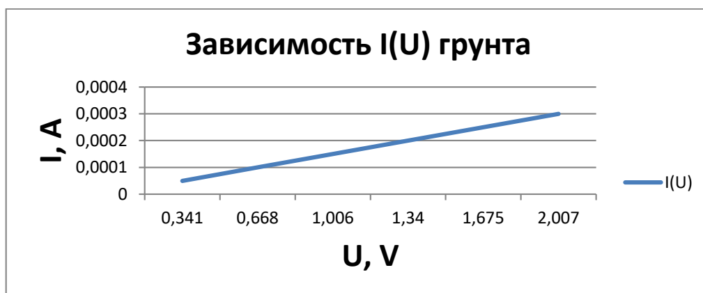
Рисунок 2 - Зависимость приложенного тока к 1 и 4 электродам от напряжения на 2 и 3 электродах (грунт)
